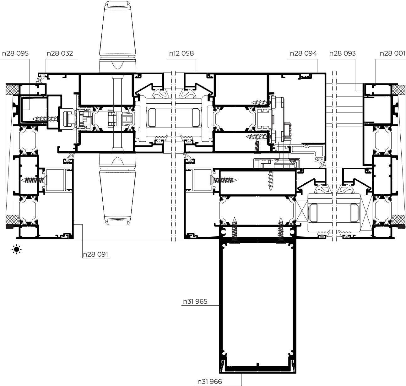
Corte C-C' Section C-C'
