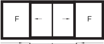
Janela deslizo batente 2 folhas + 2 fixos laterais 2 sashes open and slide window + 2 lateral fixed
