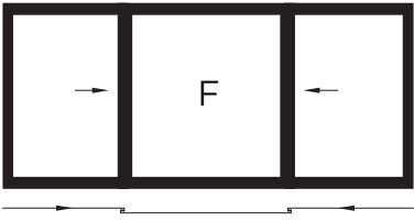
Janela deslizo batente 2 folhas + fixo 2 sashes open and slide window + fixed
