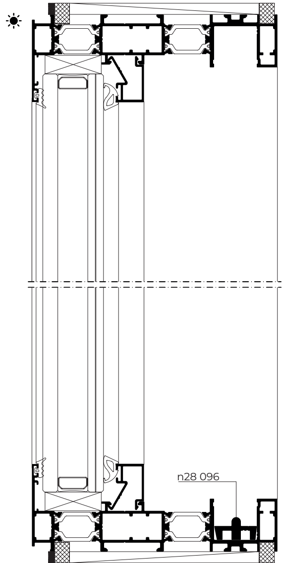
Corte B-B' Section B-B'
