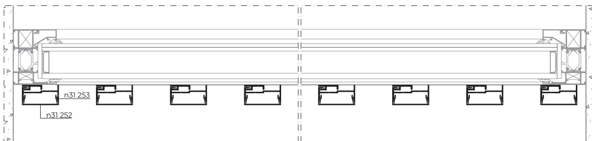
Corte B-B' Section B-B'
