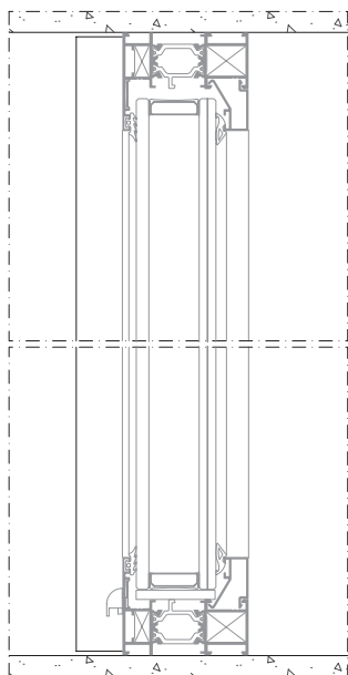
Corte A-A' Section A-A'
