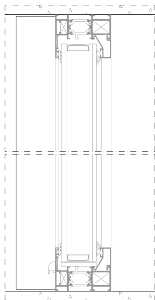
Corte A-A' Section A-A'
